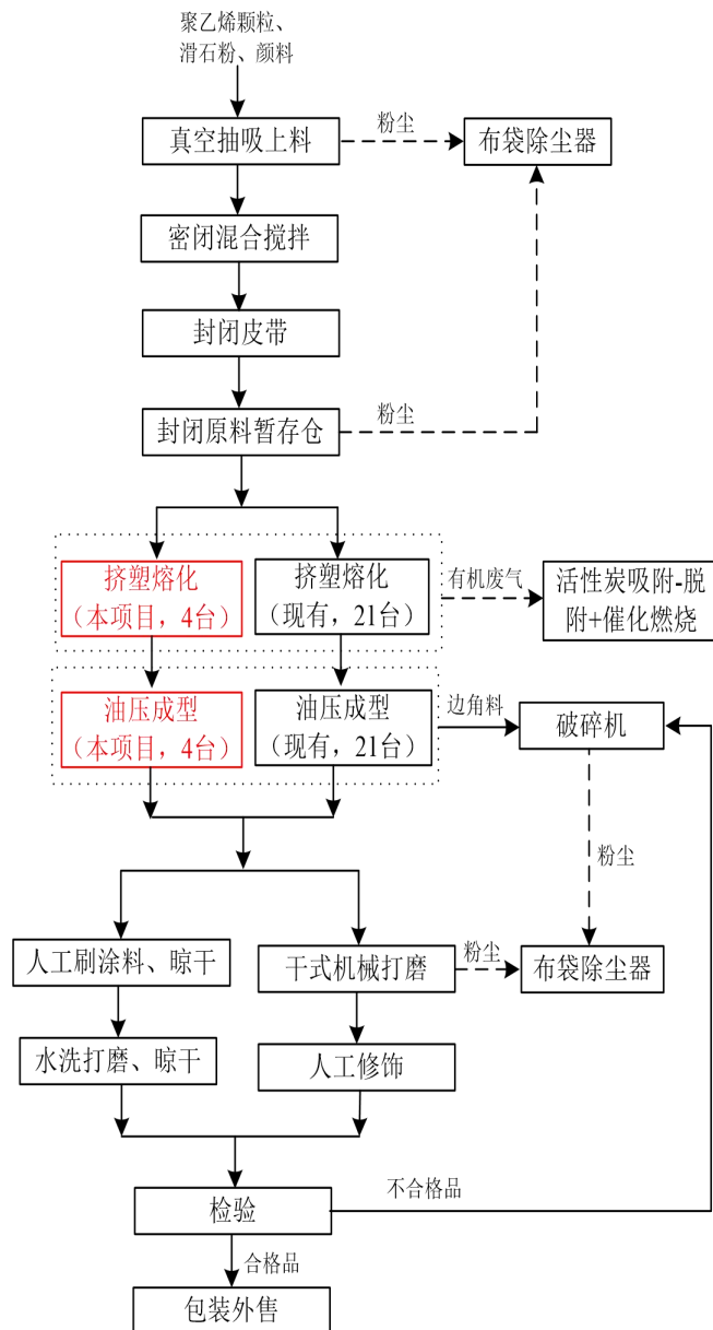
图 2.1 改建项目实施后全厂生产线工艺流程及产污环节图（红色为改建项目新增）
