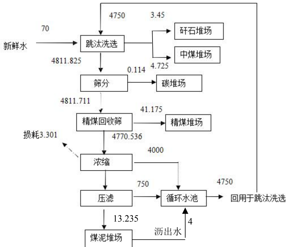
图 1 本项目水平衡图单位 m 3 /d
