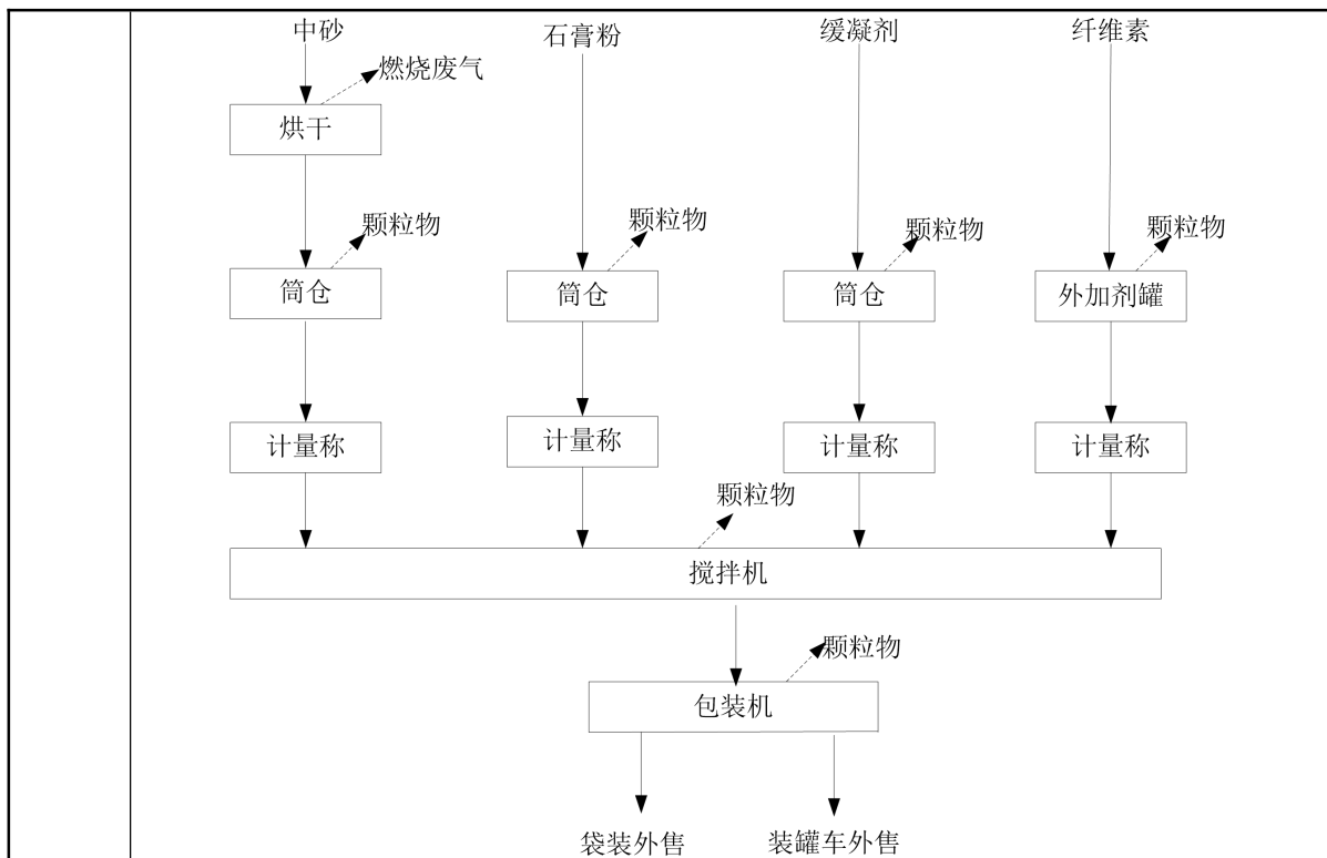
图 2.3 现有工程（干混砂浆）生产工艺及产污环节流程
