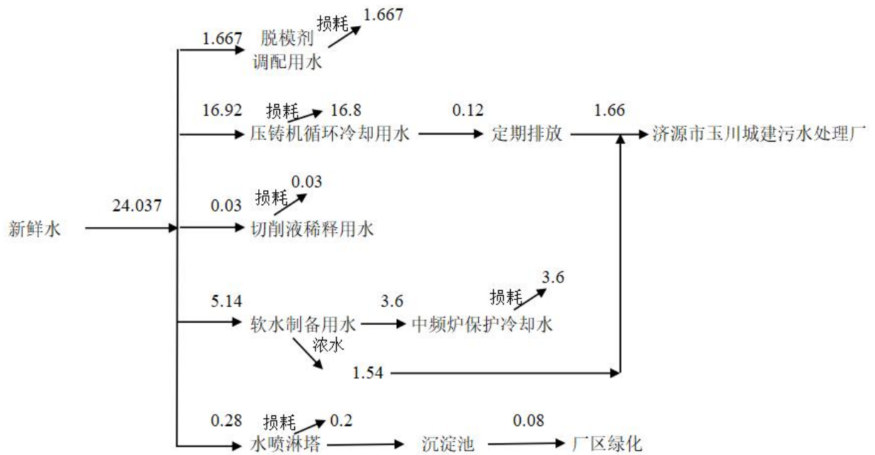
图 1 本项目水平衡图 (m³/d)
