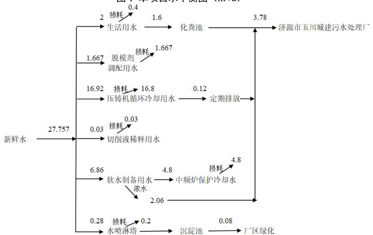
图 2 改建后全厂水平衡图
