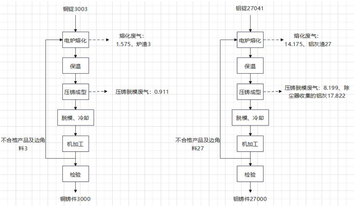
图 4 物料平衡图 (t/a)
