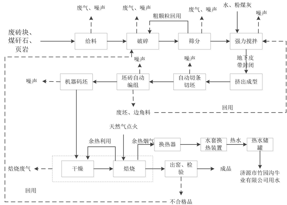
图 2-3 生产工艺流程及产污环节示意图
