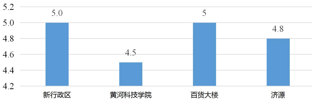
图1 济源5月份城市点位月降尘量
