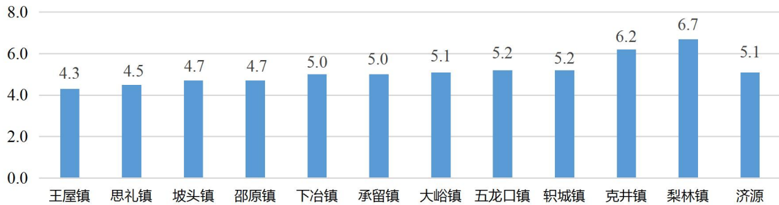
图3 2024年1-5月份乡镇降尘量平均值
