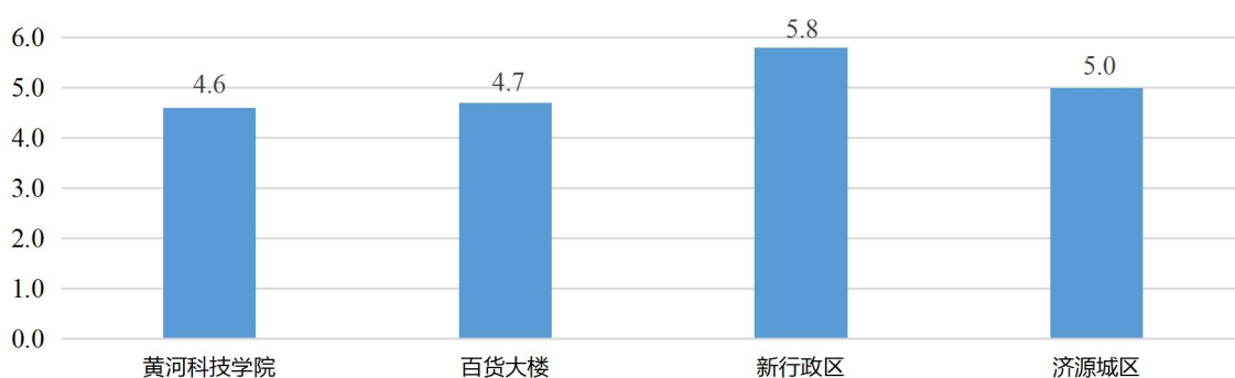
图2 2024年2-5月份城区降尘量平均值
