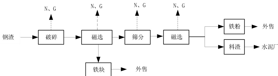
图 2 现有工程工艺流程及产污环节图
