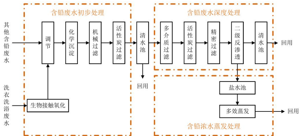
图 3 项目依托华申电源含铅废水处理站处理工艺流程示意图
