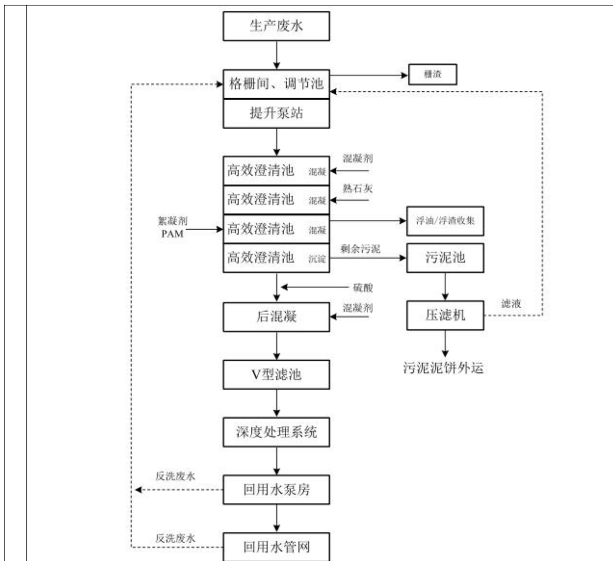
图3 企业现有污水处理工艺图
