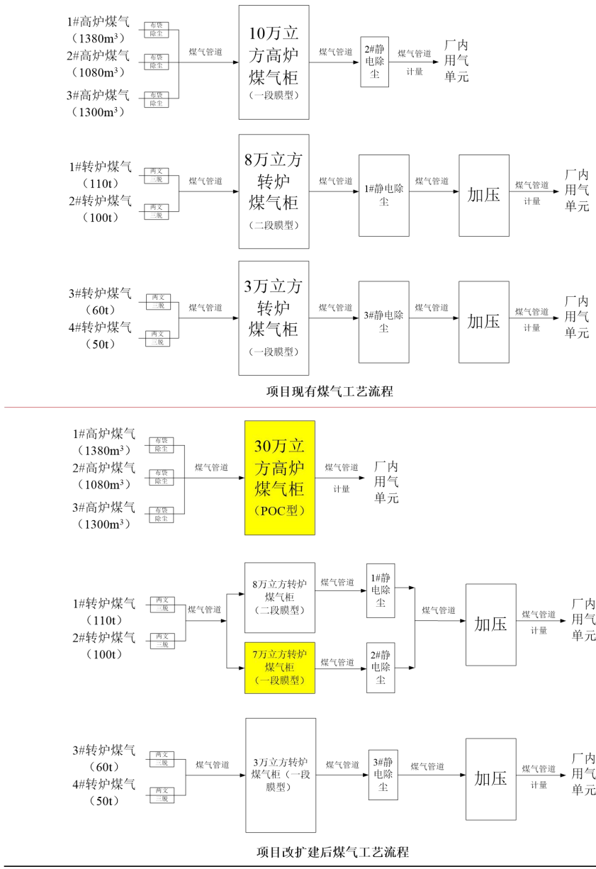
图 1 项目生产工艺流程及产污环节图
