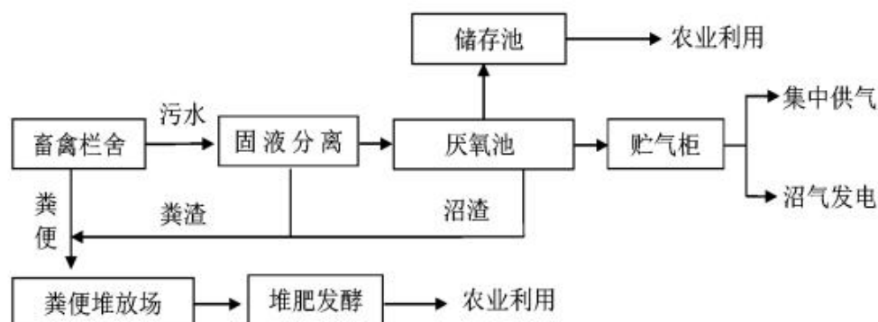
图 4 能源生态型模式工艺流程图 (方式四)
