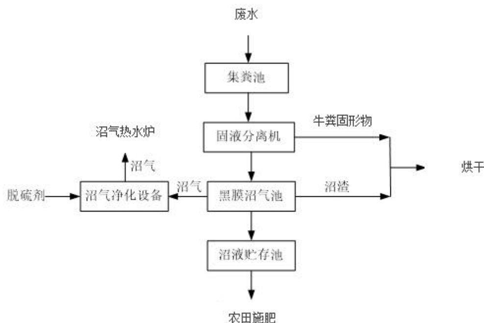
图 3-10 项目污水处理工艺流程图
