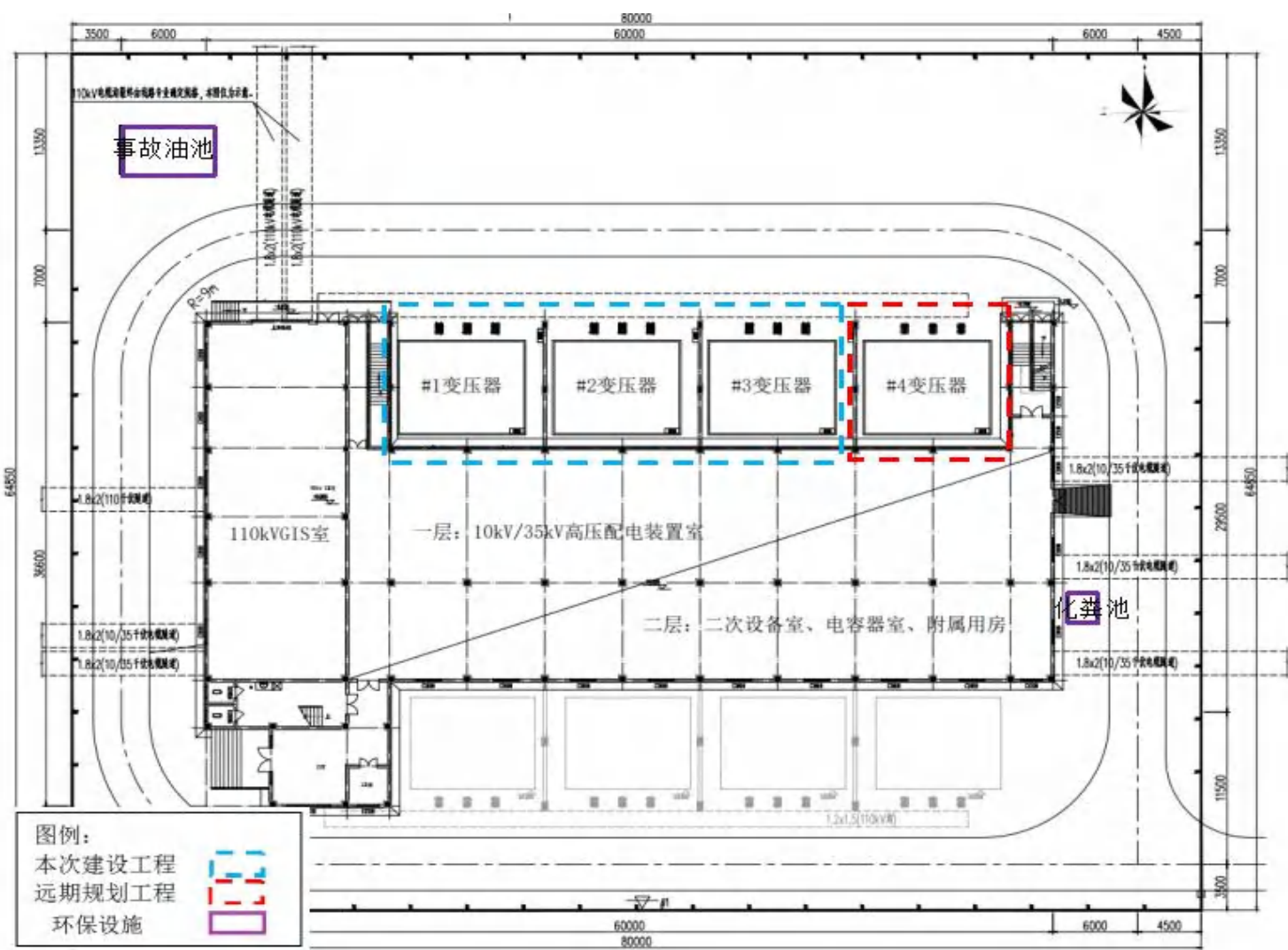
附图 5.2 本项目变电站及环保设施布置图
