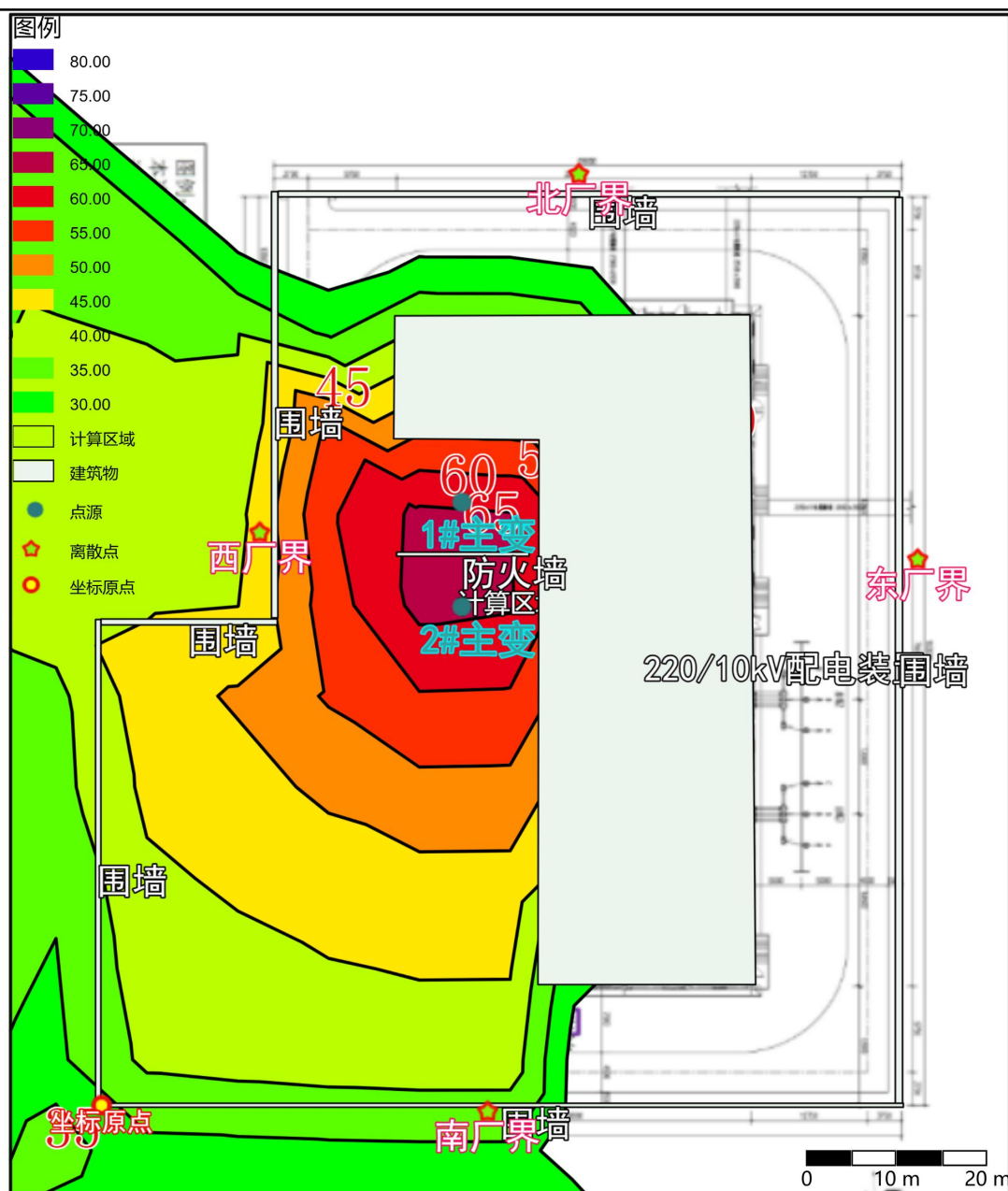
图4-3 项目远期噪声贡献值等声级线分布图
