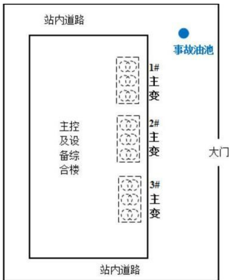
专图 3 类比站人民 220kV 变电站变电站平面布置图
