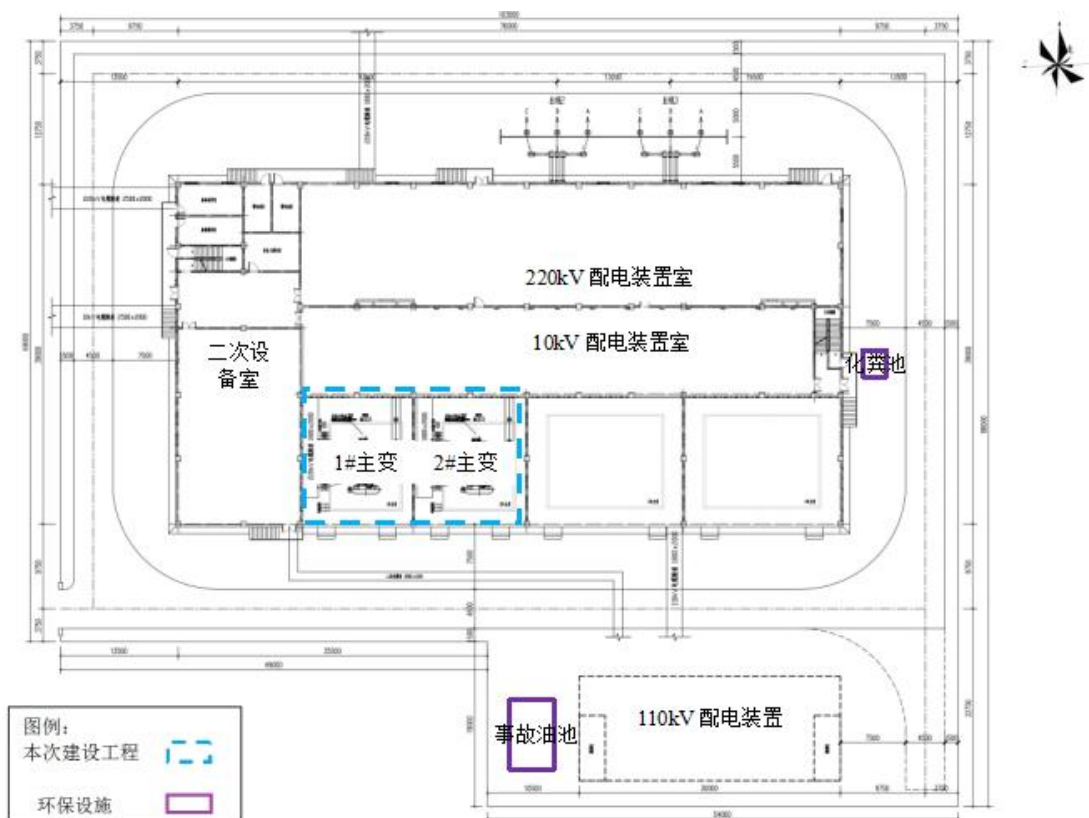
专图 2 锌业 220kV 变电站平面布置图
