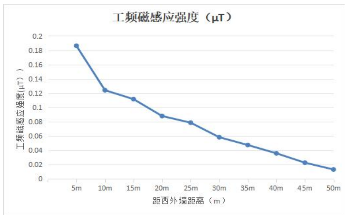
专图 6 类比 220kV 变电站围墙外工频磁感应强度衰减趋势图
