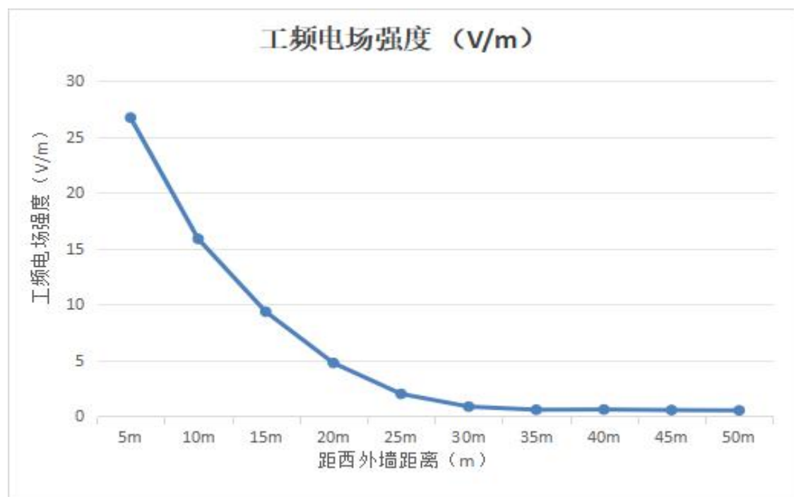
专图 5 类比站 220kV 变电围墙外工频电场强度衰减趋势图
