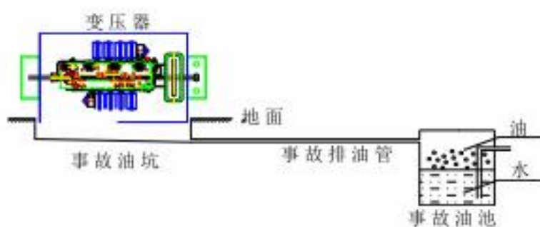
图 4-4 事故油坑、事故排管道及事故油池布置平面图（参照同类型布置）
