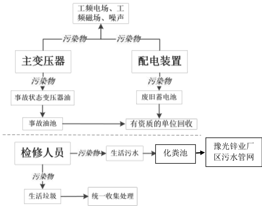
图4-2 工程运行期主要产污环节示意图
