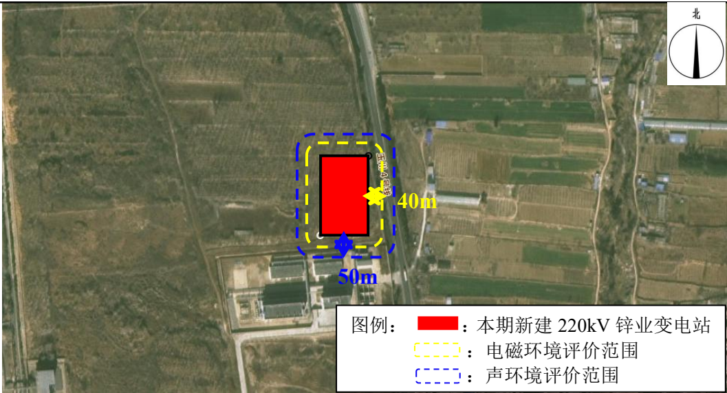
图 3-4 新建锌业 220kV 变电站电磁环境和声环境评价范围示意图
