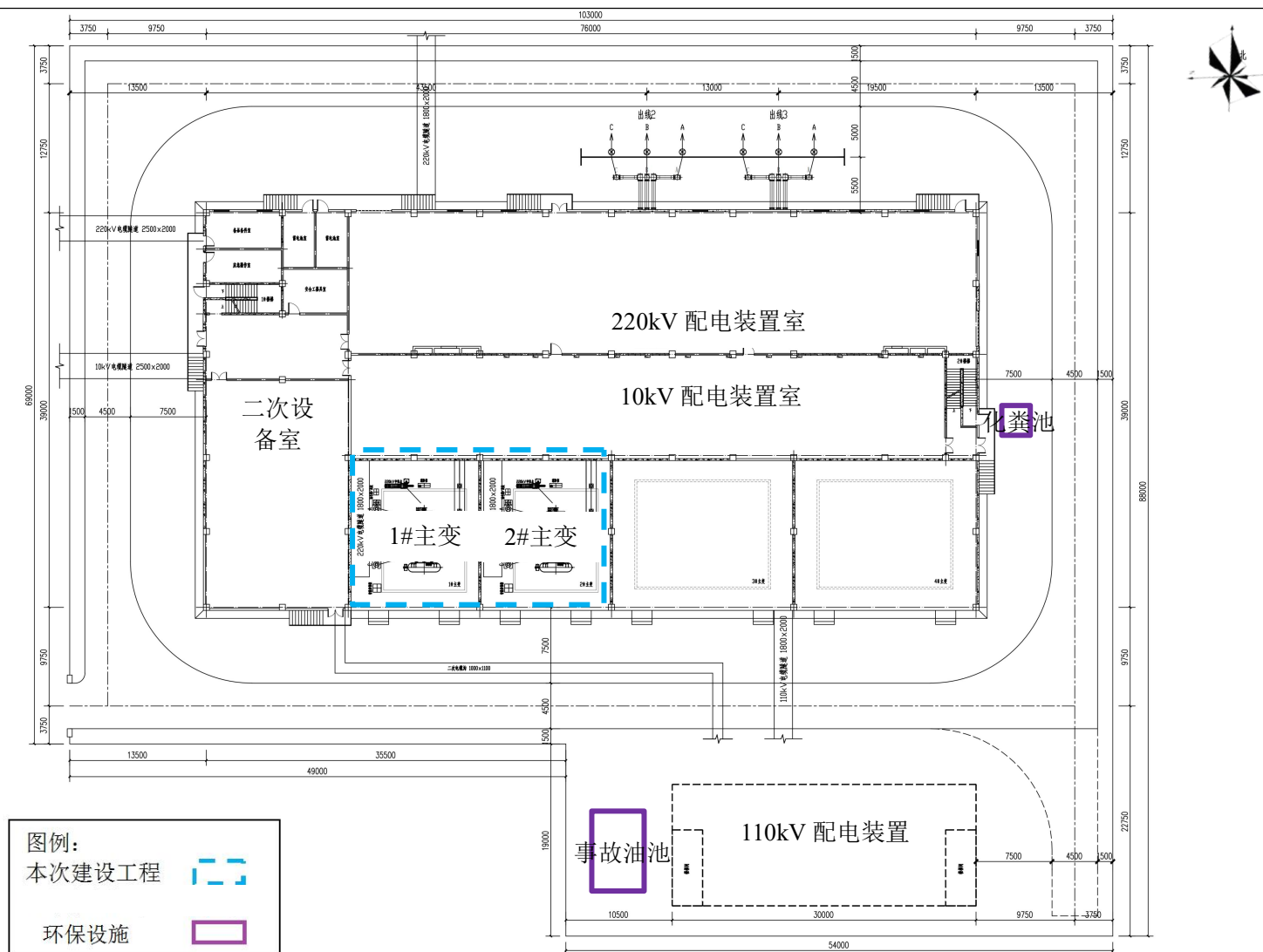
图2-2 变电站平面布置图
