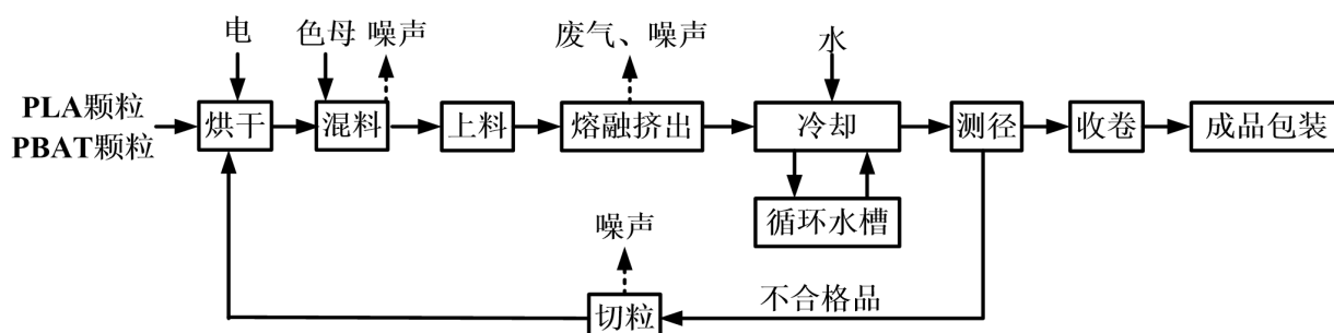
图 2.2 项目工艺流程及产污环节图
