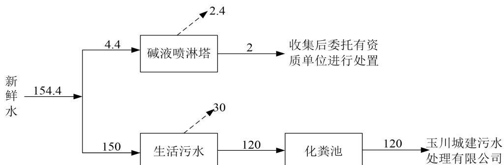
图 2.1 本项目水平衡图 单位： \text{m}^3/\text{a}
