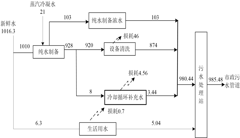
图 2-1 改建项目水平衡 单位：m³/d
